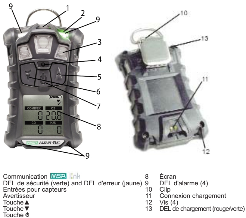
Figure 2-1. Aperçu de l'appareil
